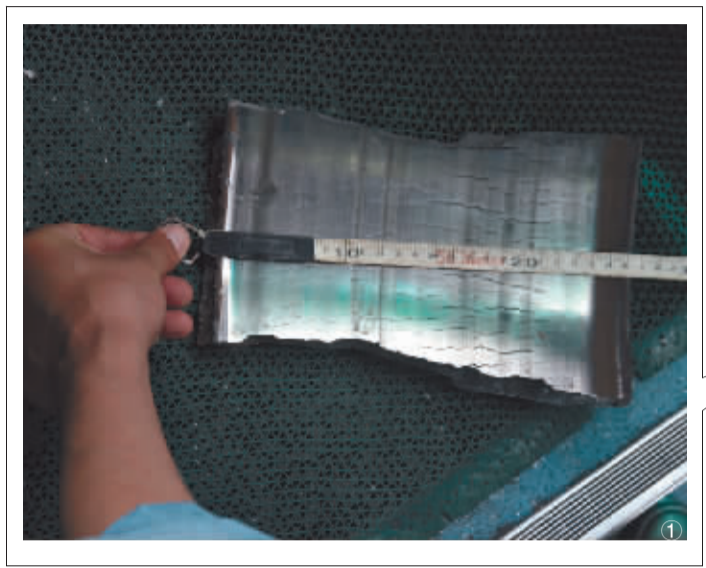
图①为警方提供的造成吴斌死亡的制动毂脱落残片照片。 图②为警方提供的肇事车辆照片。
